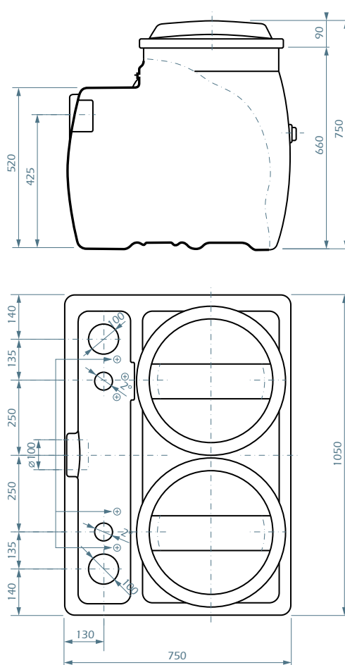
ENCOMBREMENTS 2 POMPES
