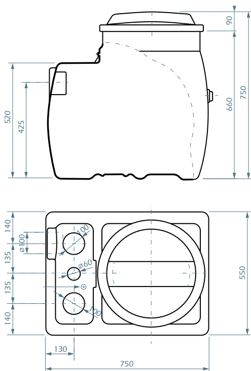
ENCOMBREMENTS 1 POMPE
